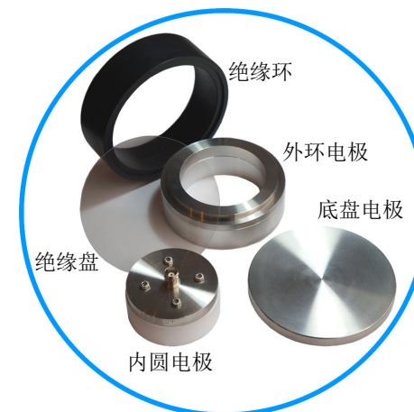
TE50 电极分解图
