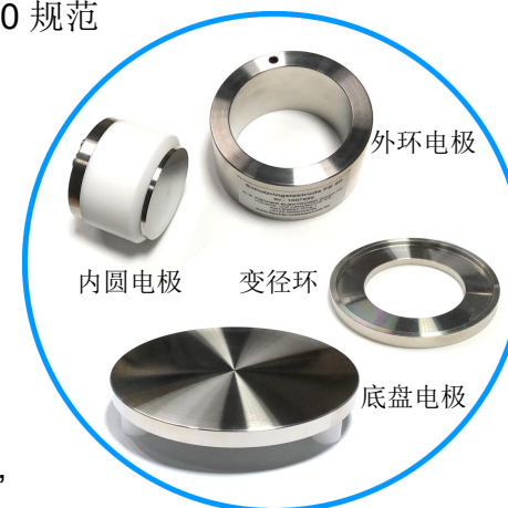
FE50 电极分解图
